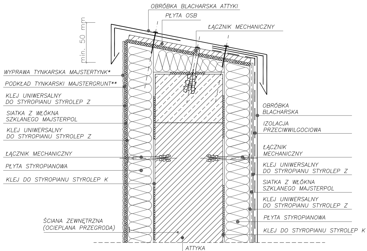
DETAL OCIEPLENIA ATTYKI PRZEKRÓJ PIONOWY
