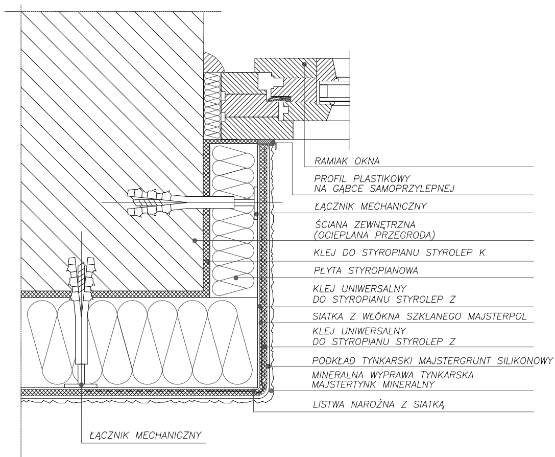
DETAL OCIEPLENIA OSCIEŻA PRZEKRÓJ POZIOMY
