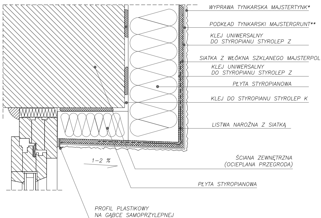
DETAL OCIEPLENIA NADPROŻA OKIENNEGO I DRZWIOWEGO PRZEKRÓJ PIONOWY
