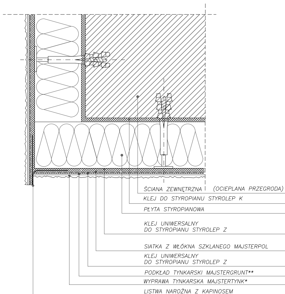
DETAL OCIEPLENIA NAROŻA PODCIENIA PRZEKRÓJ POZIOMY
