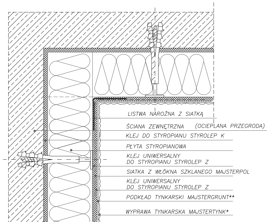
DETAL OCIEPLENIA NAROŻA WKŁĘŚŁEGO PRZEKRÓJ POZIOMY
